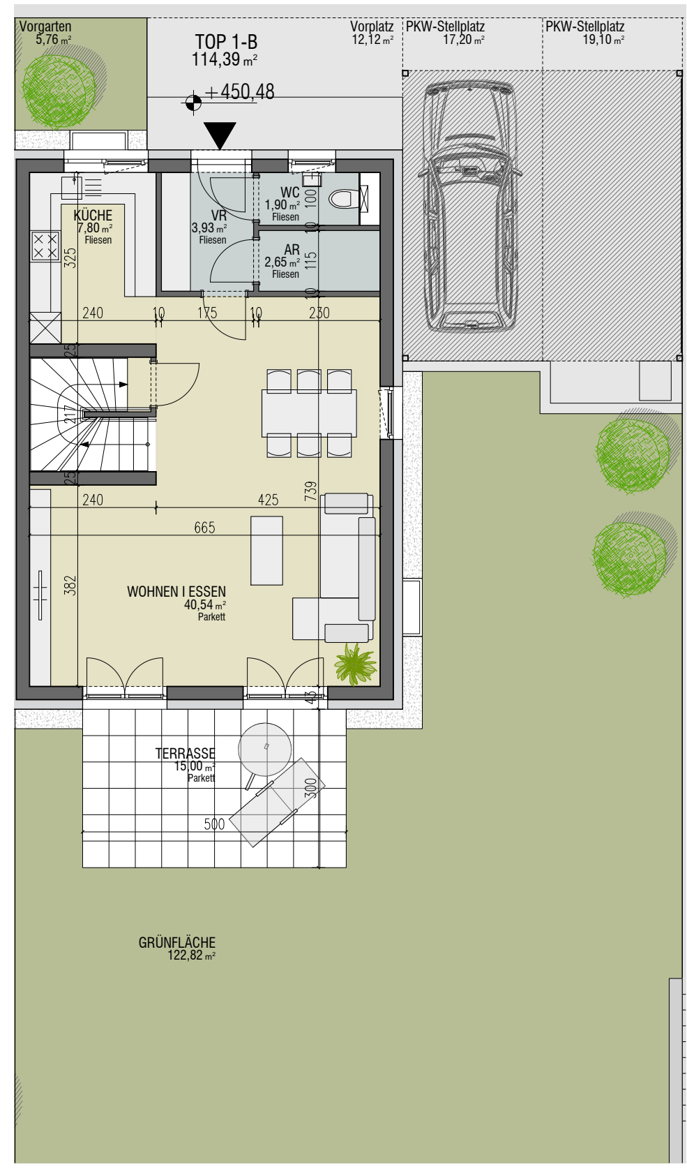
ERDGESCHOSS
