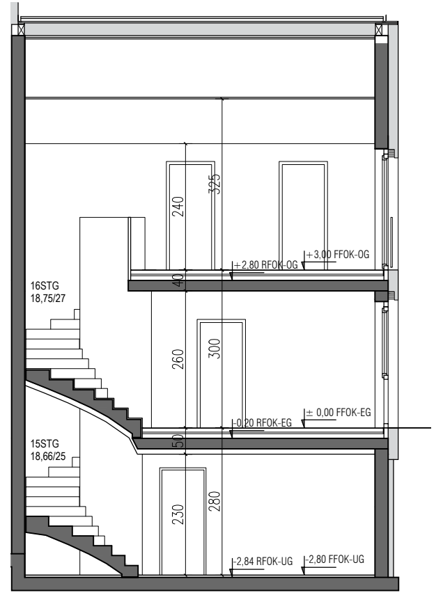
SYSTEMSCHNITT
