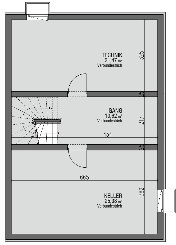
KELLERGESCHOSS
