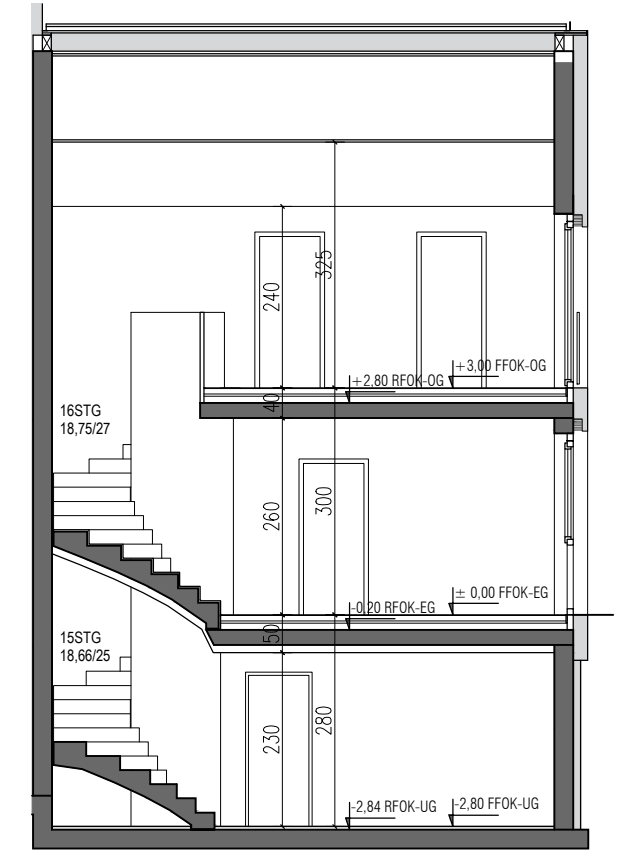
SYSTEMSCHNITT
