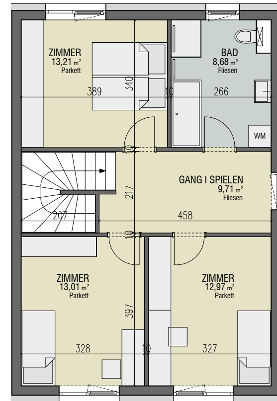
OBERGESCHOSS
