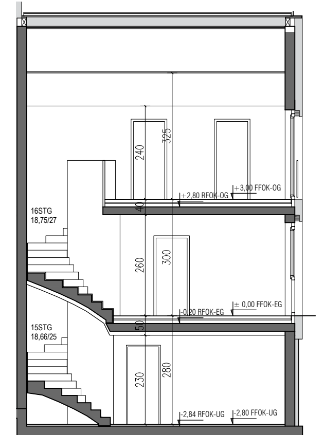
SYSTEMSCHNITT
