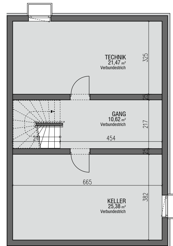
KELLERGESCHOSS
